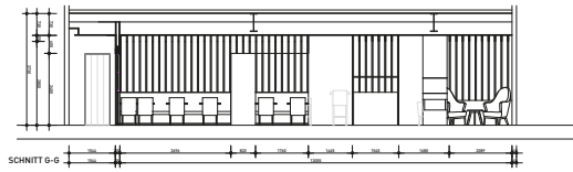
SCHNITT G-G
