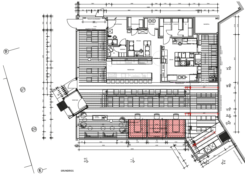
GRUNDRISS
