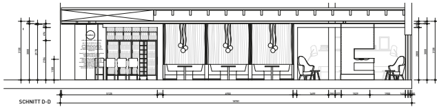
SCHNITT D-D
